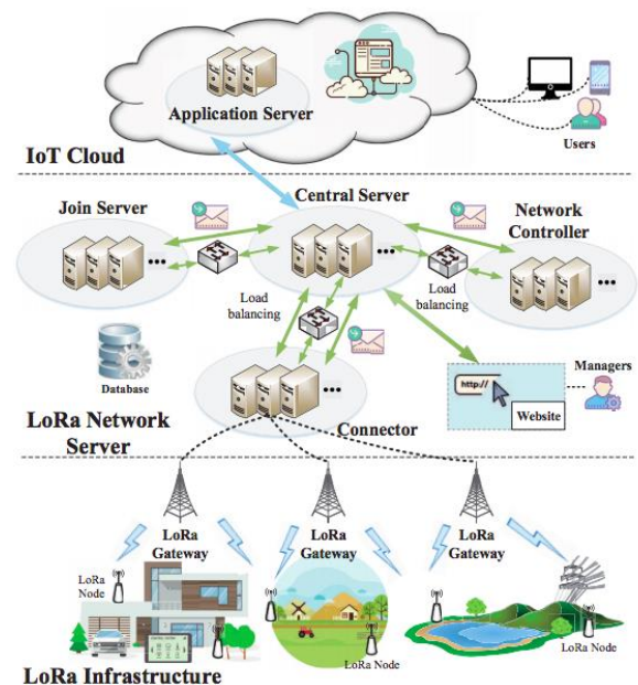
Hình 3 Cấu trúc của mạng LoRa [6]
