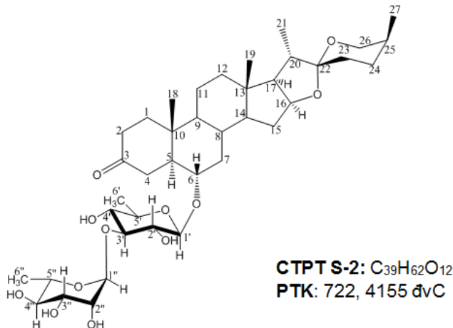
Hình 3 Cấu trúc và những tương tác trong cấu trúc hóa học hợp chất S-2
