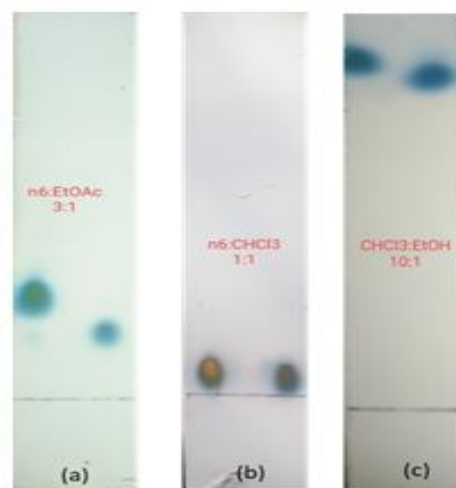
Hình 2 Kết quả sắc kí lớp mỏng 2 phân đoạn thu được (a) hệ n -hexan:ethyl acetat = 3:1; (b) hệ n -hexan:chloroform = 1:1; (c) hệ chloroform:ethanol = 10:1 (phân đoạn 1 bên trái và phân đoạn 2 bên phải)
