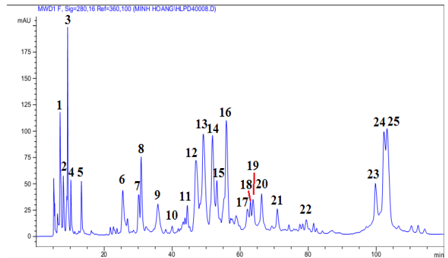
Hình 4. Sắc ký lỏng cao áp trên cột C18 của nọc bò cạp Heterometrus laoticus
